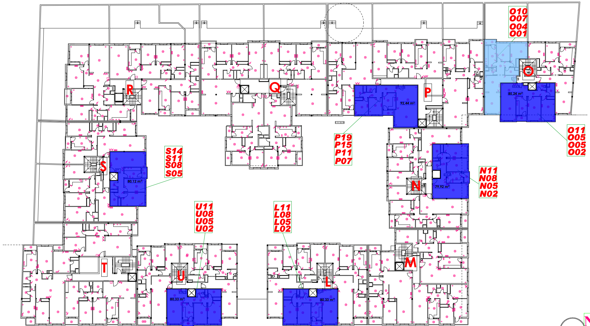
PLAN ETAGE COURANT 1 er -2 eme -3 eme ET 4 eme ETAGES
